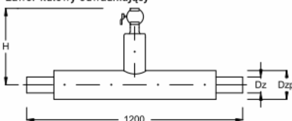
Zawór kulowy odwadniający
